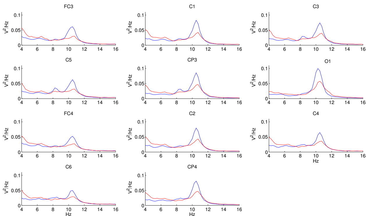
Obr. 2: Porovnanie normalizovaného výkonového spektra pre jednotlivé dni u vybraného zdravého subjektu (muž, 28 rokov) počas relaxácie so zatvorenými očami pred začiatkom (modrá krivka) a po skončení (červená krivka) motorického cvičenia so zrkadlovým boxom. Hodnoty spektrálneho výkonu boli odhadnuté FFT metódou na 4-sekundových segmentoch EEG, normalizované celkovým výkonom v pásme 4–30 Hz a následne spriemernené (pozri text).
